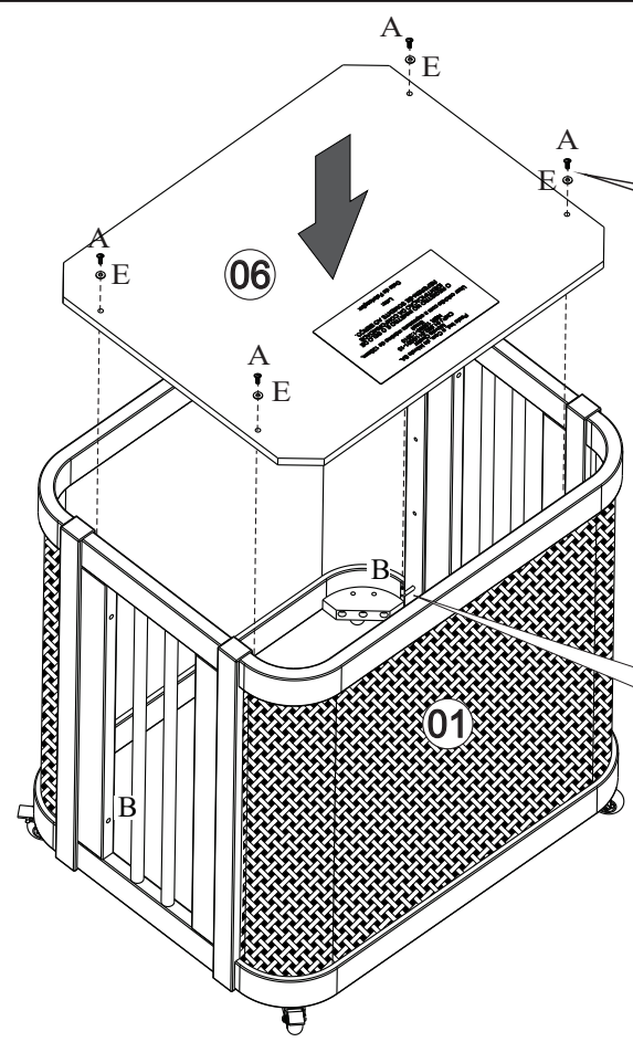
Fixação do estrado lado direito
